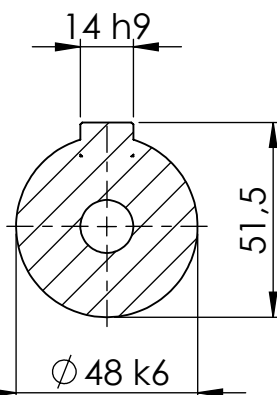
SECTION A-A SCALE 1 : 2
