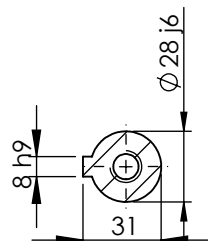
SECTION A-A SCALE 1 : 3
